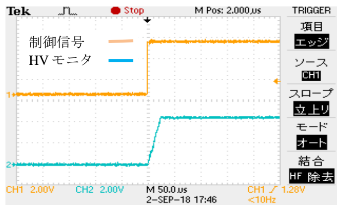
図2. 有負荷立ち上がり特性 (1.8 μF の場合)
