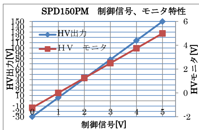
図1. 入出力特性
